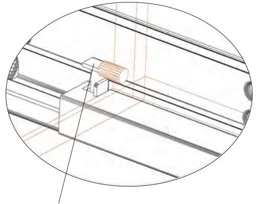
FERMO POSTERIORE DEL CASSETTO A GUIDA MONTATA POSTERIOR DETENTION OF THE DRAWER TO MOUNTED SLIDE ARRÊT POSTÉRIEUR DU TIROIR Á GLISSIÈRE MONTÉE HINTERE VERZÖGERUNG DES FACHES ZU ANGEBRACHTEM FÜHRER DETENCIÓN POSTERIOR DEL CAJON A LA GUÍA MONTADA
